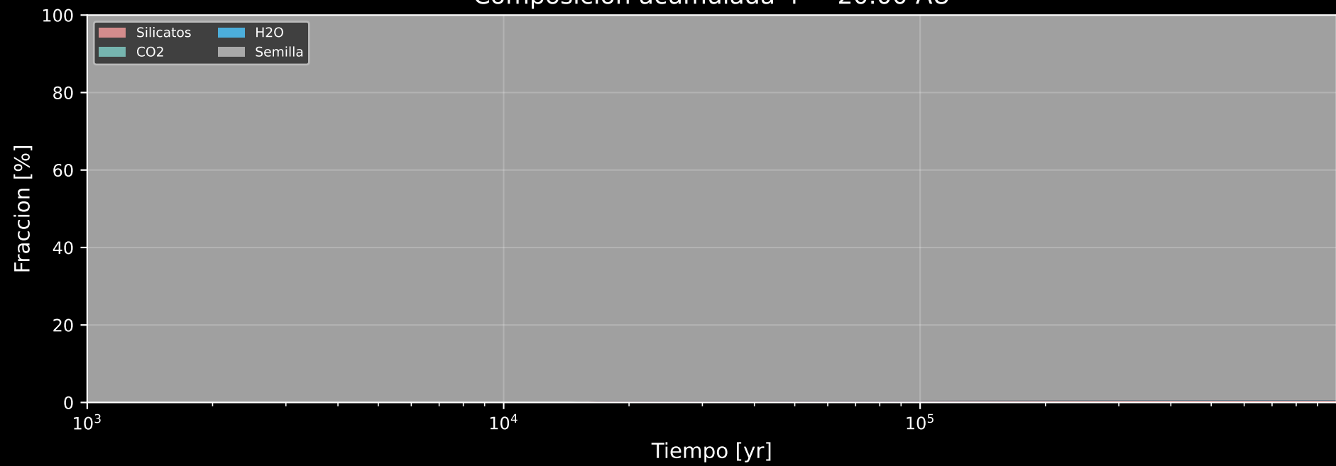
Composicion acumulada r = 20.00 AU
